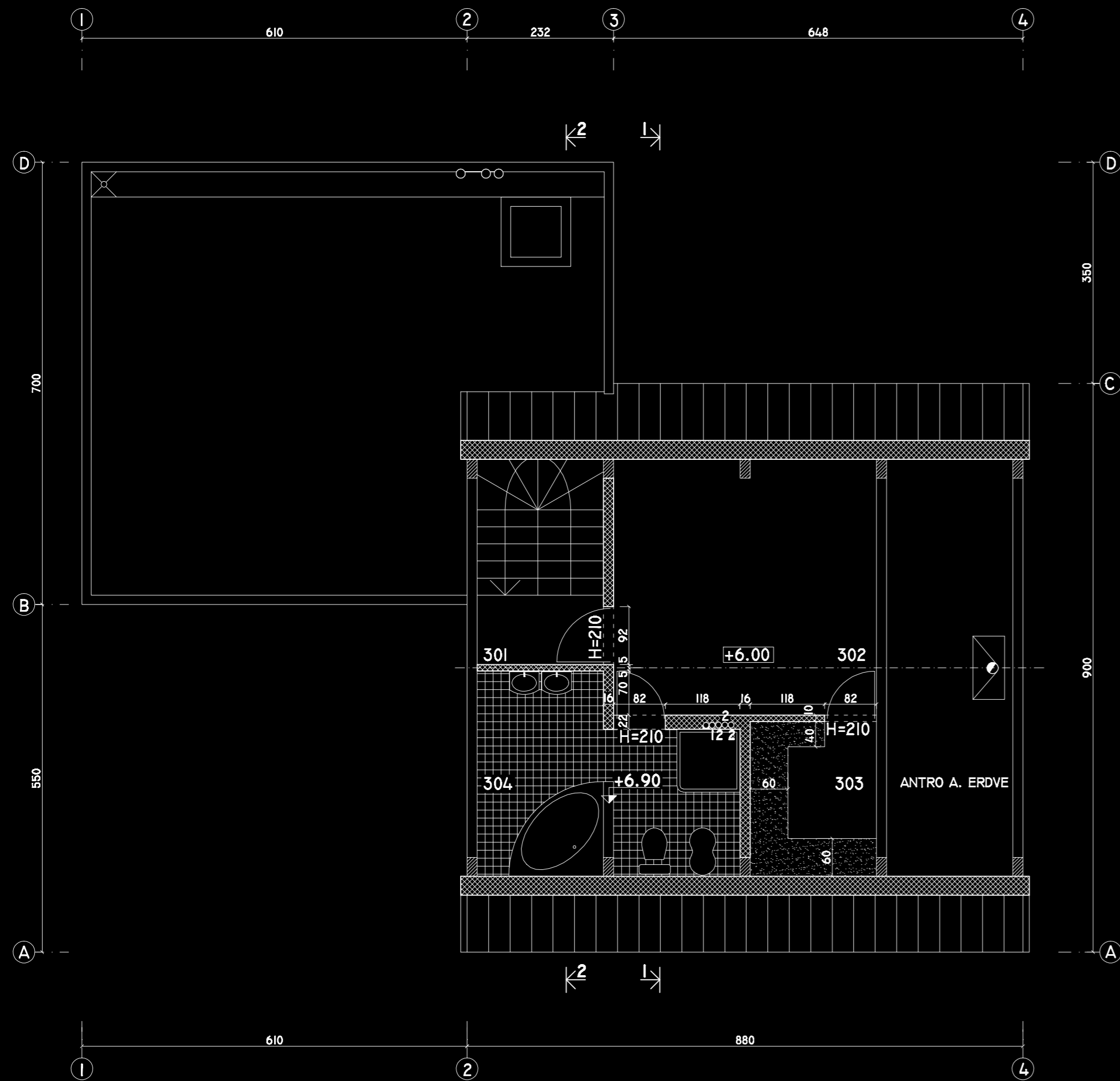
TRECIO AUKSTO PLANAS M 1:100
