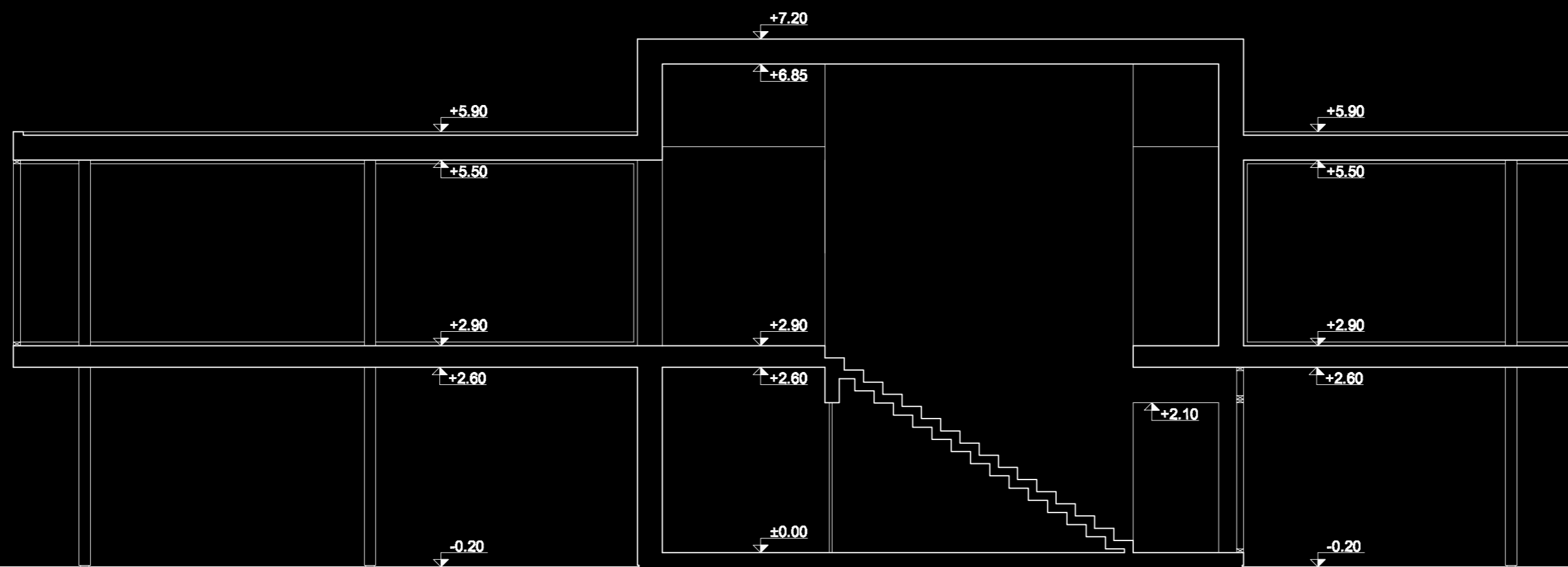
PJŪVIS 2-2 M 1:100
